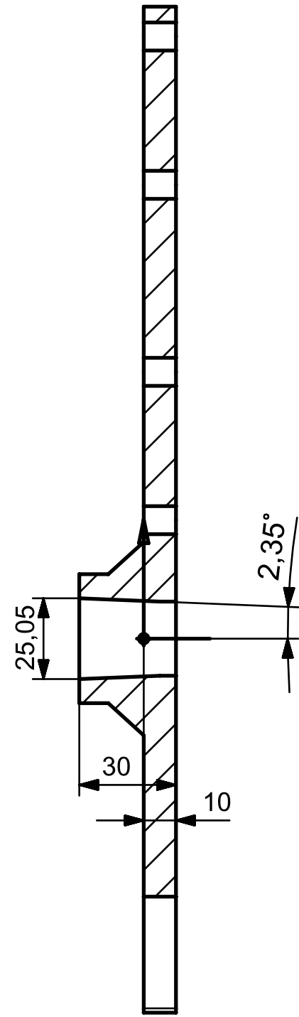
SECTION A-A
